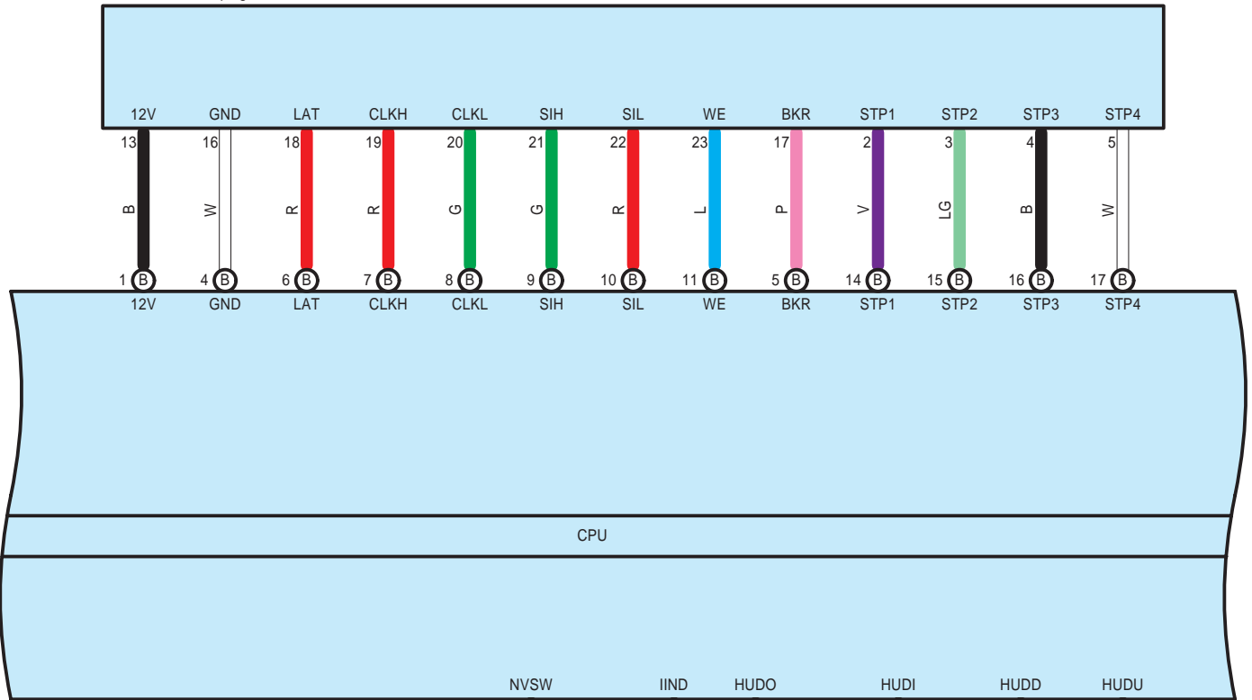
L27(A), L106(B), L107(C) Kombiinstrument-Baugruppe
